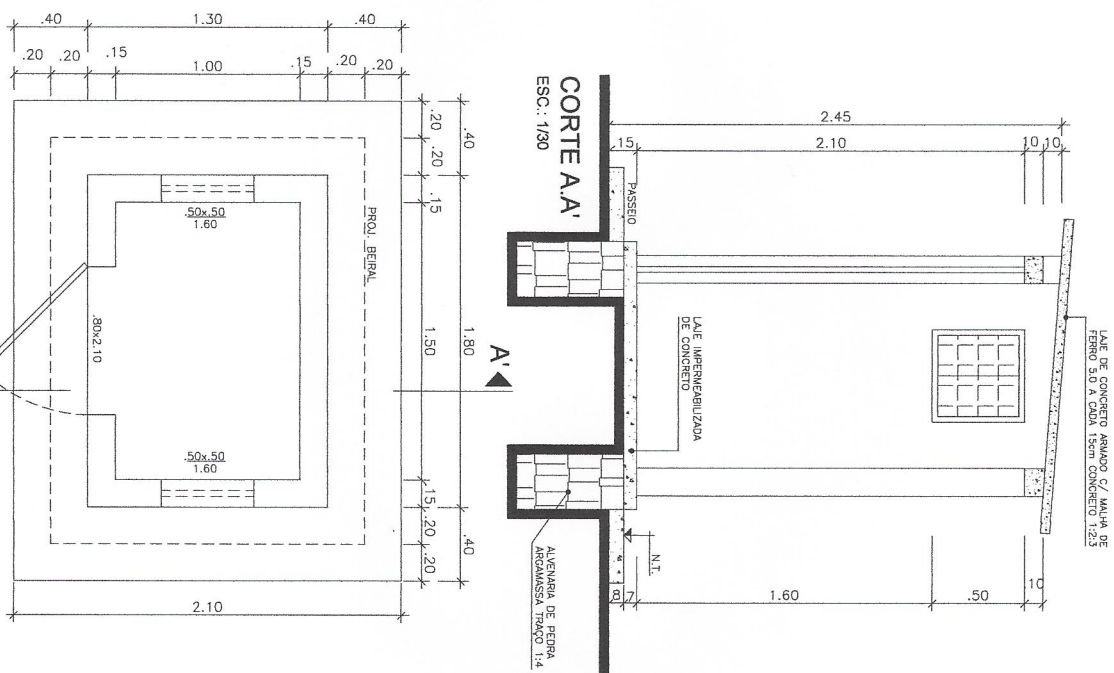
PLANTA BIAXA ESC.: 1/30
